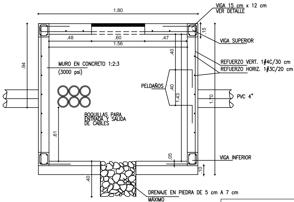
SECCIÓN DE RECÁMARA
