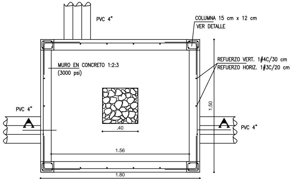
PLANTA DE RECÁMARA
