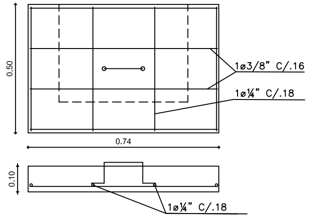
DETALLE DE TAPA
