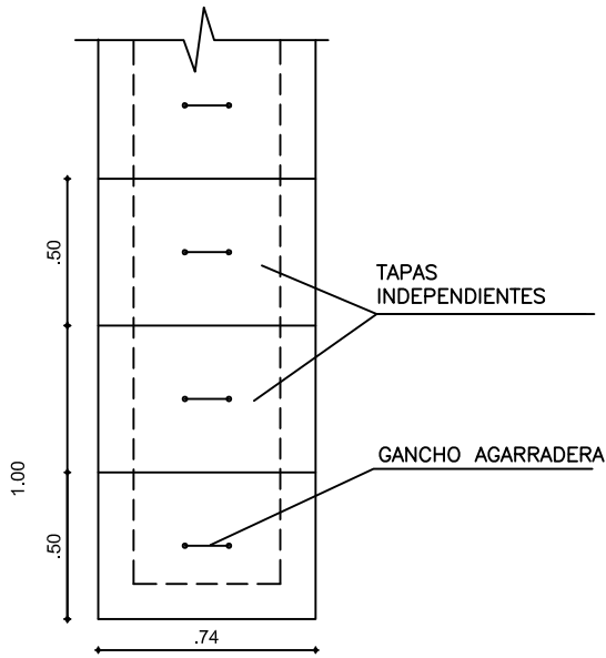
DETALLE DE TAPA
