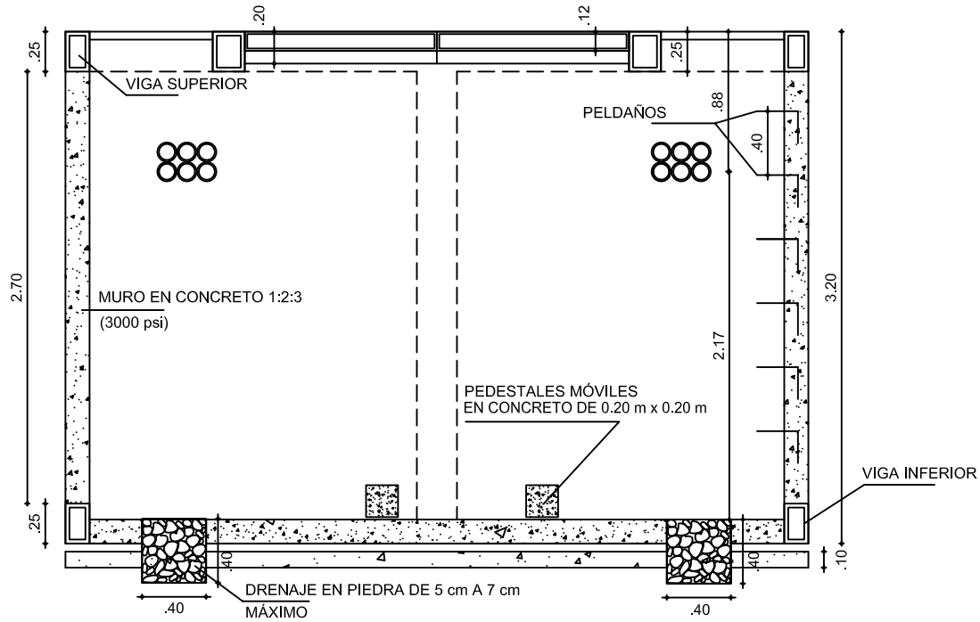
SECCIÓN LONGITUDINAL
