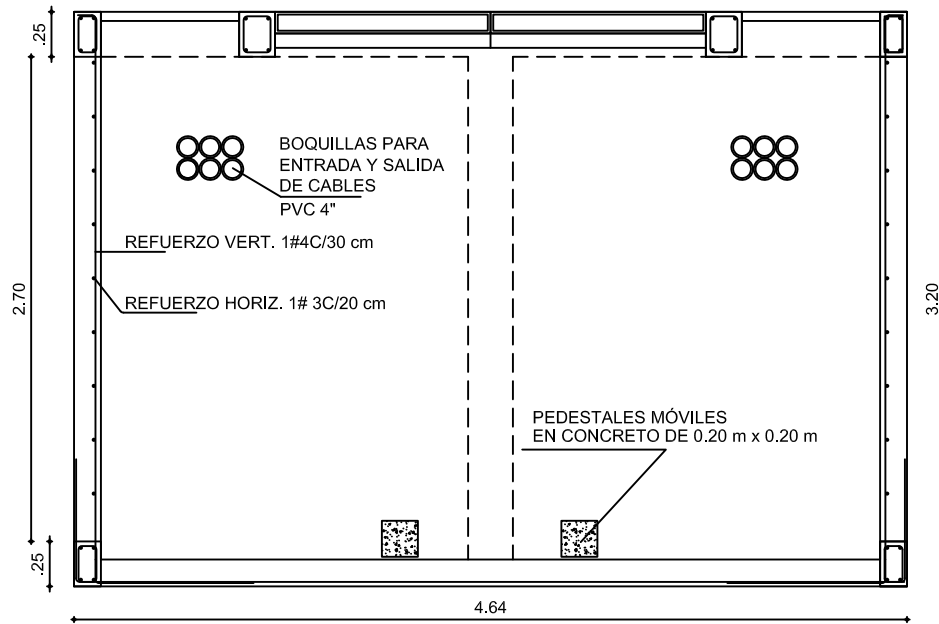
SECCIÓN LONGITUDINAL
