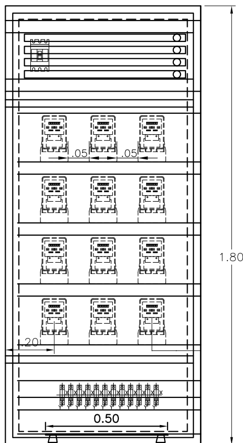
12 CUENTAS 0.80 VISTA FRONTAL SIN PUERTAS
