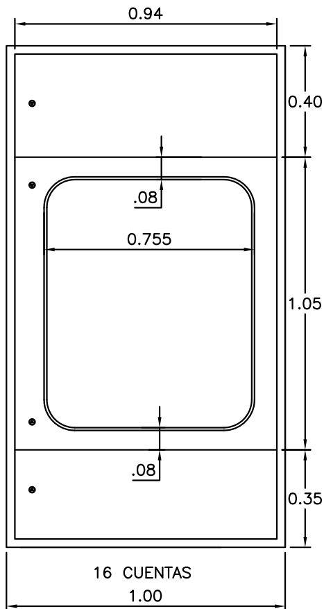
VISTA FRONTAL CON PUERTAS
