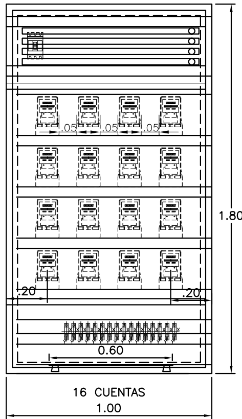
VISTA FRONTAL SIN PUERTAS
