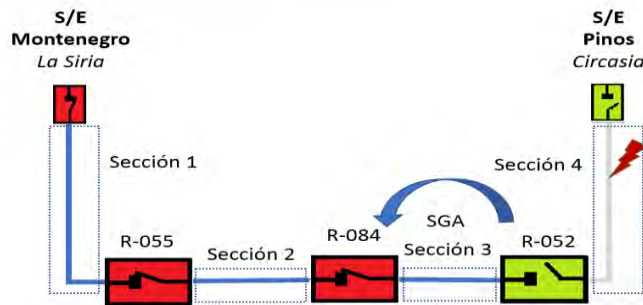
Fig. 5. Falla permanente Sección 4.
