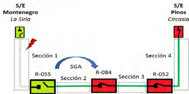
Fig. 4. Falla permanente Sección 1
