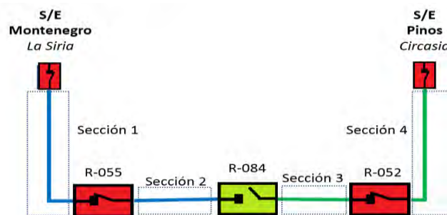
Fig. 3. Secciones de operación
