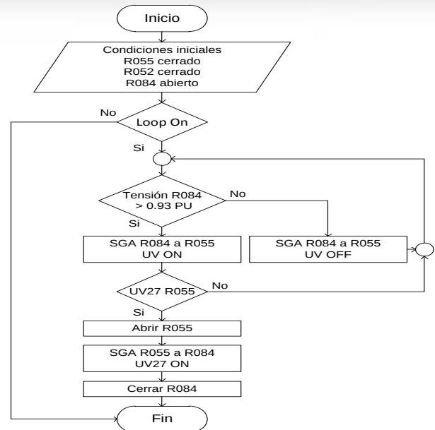
Fig. 6. Diagrama de flujo SGA
