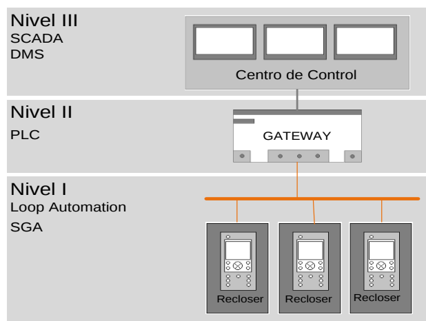
Fig. 1. Niveles de automatización definidos en EDEQ SA ESP
